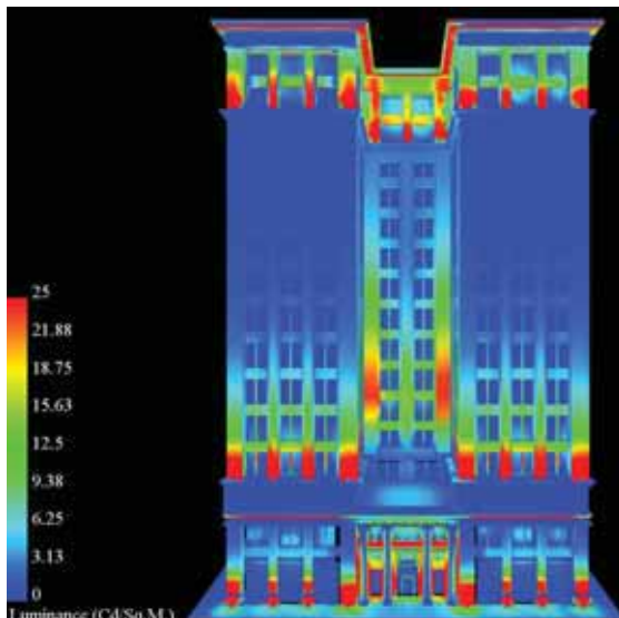
Figura 3 Luminância da fachada de um edifício. Nas áreas vermelhas este parâmetro excede o valor de 25 cd/m 2 .
