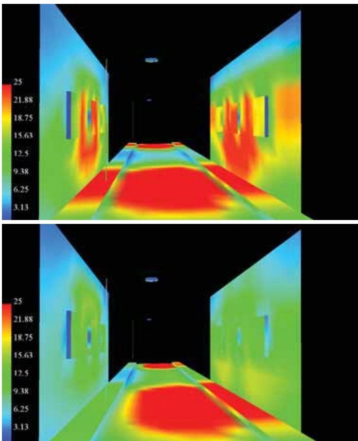
Figura 2 Invasão de luz produzida por unidades de iluminação pública. Flagrante de um caso real e simulações com dois tipos de luminárias. Na última simulação, a luminária utilizada não infringe os limites estabelecidos pela Publicação CIE 150:2003 para o limite de 25 lx.
